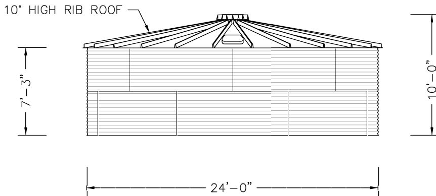
ELEVATION
